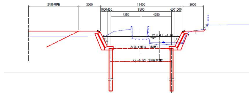
善太川改修断面図
